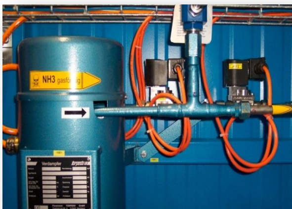
Verdampfer
